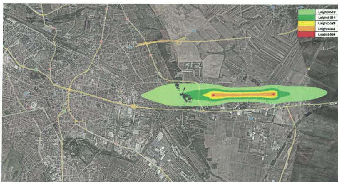
Figura 3. Harta de zgomot L_{noapte} Aeroportul Internațional Craiova (2021)
